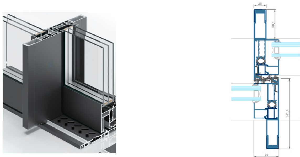
SECCIÓN CRUCE REDUCIDO
