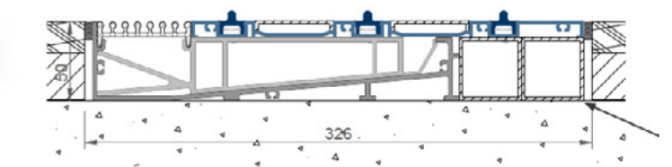
SECCIÓN RECOGIDA DE AGUA 3 CARRILES THERMIA LEVITA
