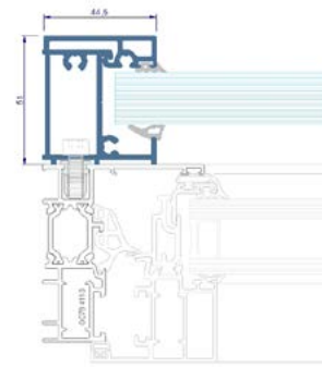
PARTIE LATÉRALE INTÉGRÉE AVEC SYSTÈME THERMIA LUMIA OC78
