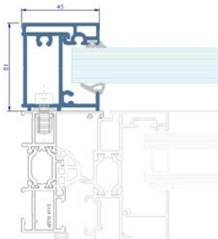
PARTIE LATÉRALE INTÉGRÉE AVEC SYSTÈME THERMIA HABITAT AR78
