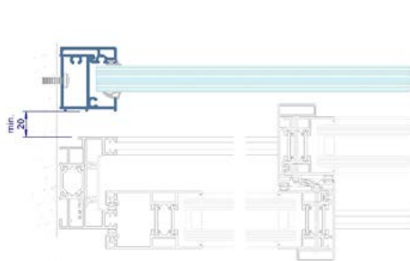
SECTION LATÉRALE AVEC SYSTÈME COULISSANT THERMIA MAGNA CR46
