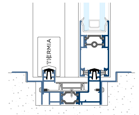
DORMANT ENCASTRÉ
