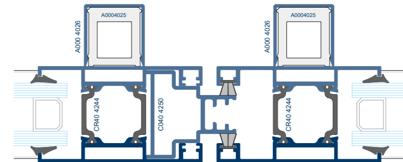
SECTION D'UN OUVRANT À FERMETURE CENTRALE RENFORCÉE
