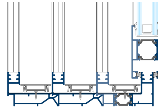
SECTION LATÉRALE MULTIRAIL
