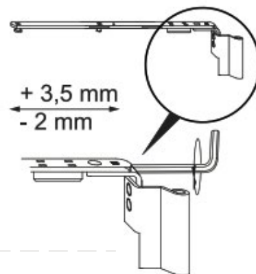
Regulación en altura de hoja (-2 hasta +3.5 mm)
