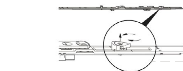
Cierre progresivo del compás. Regula de 18 a 28 mm
