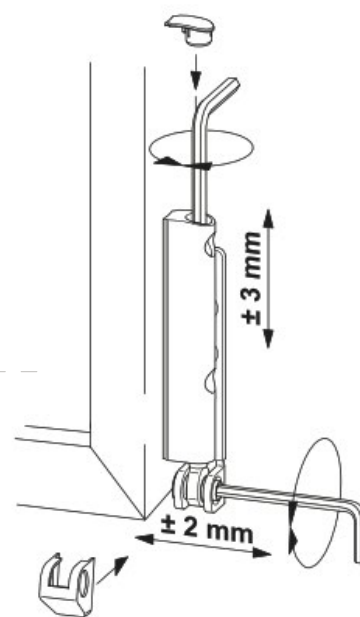
Reg. Altura ±3 mm
