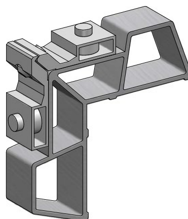
A000 2114 escuadra hoja p.
