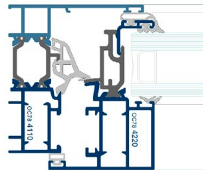
SECCIÓN LATERAL
