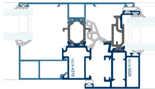
SECCIÓN CENTRAL
