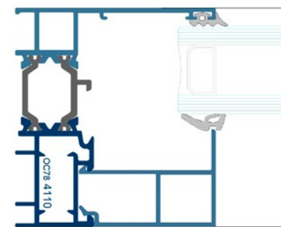
SECCIÓN LATERAL MARCO FIJO
