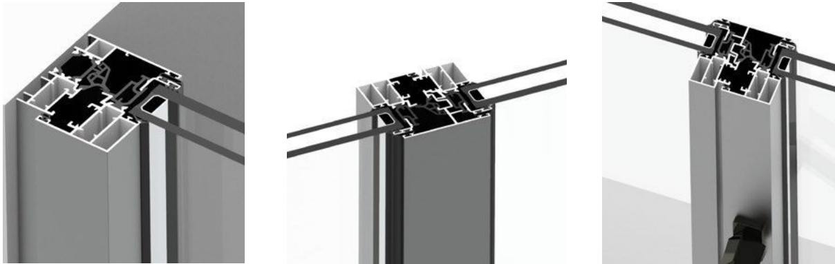
Marco lateral con hoja
