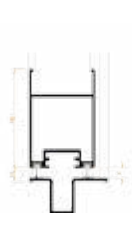
Guía inferior empotrada
