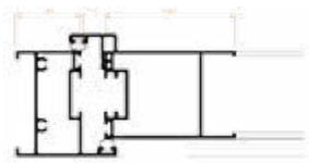
Sección 1 hoja
