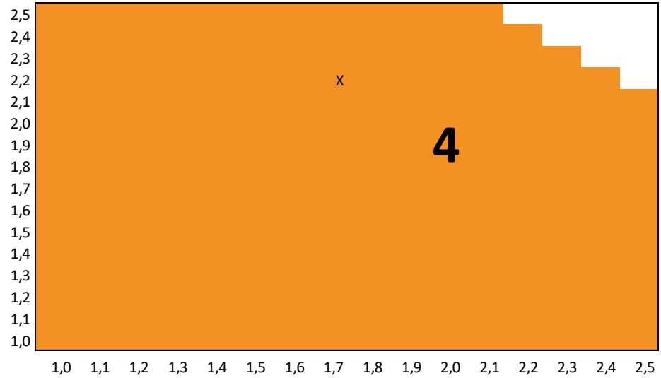
PERMEABILIDAD AL AIRE según EN 12207 - Mercado CE según EN 14351-1:2006 (E.1)
