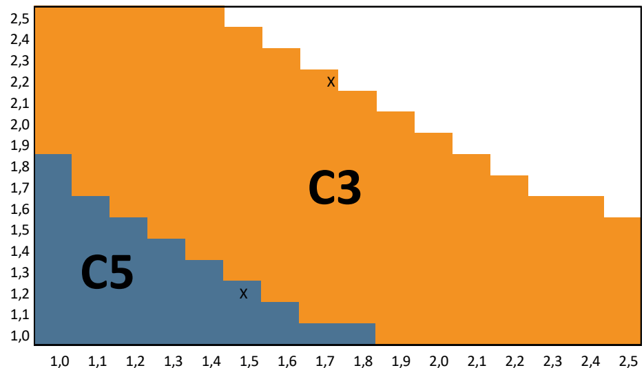
RESISTENCIA AL VIENTO según EN 12210 - Mercado CE según EN 14351-1:2006 (E.1)
