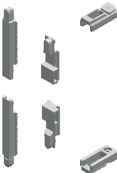
A0003110 kit accesorios hoja activa practicable (sin cremona ni bisagras)
