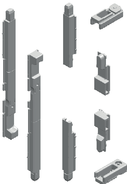
A0003112 kit accesorios dos hojas practicable (sin cremona ni bisagras)
