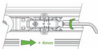
Ajuste fuga superior compás
