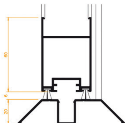
Guía inferior superpuesta
