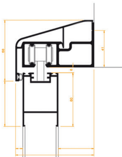
Guía pared con tapa embellecedora
