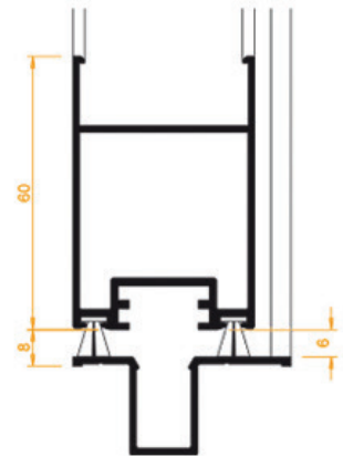
Guía inferior empotrada
