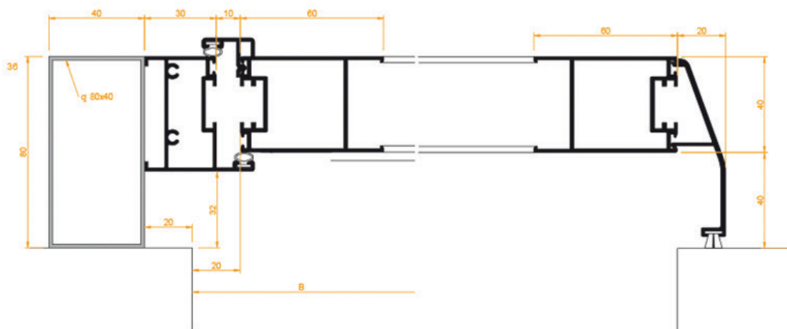
Sección 1 hoja
