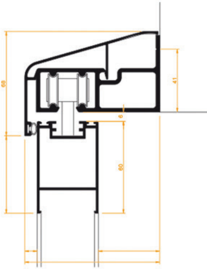
Guía pared con tapa embellecedora
