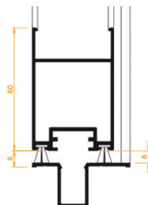
Guía inferior empotrada
