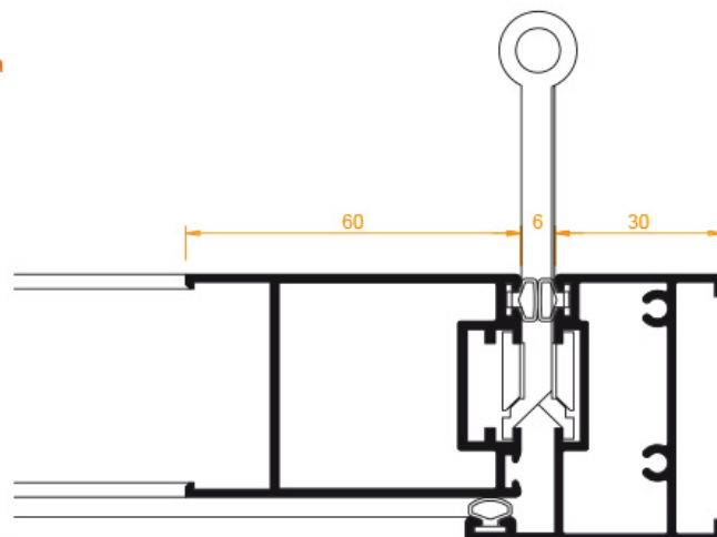
Sección 1 hoja
